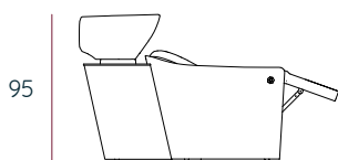
Poltrona Lavaggio | Shampoo Bowl Cm 78 x 168 x 95 h.
